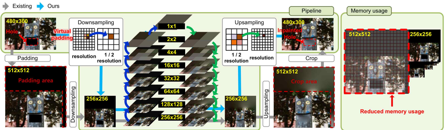
그림 1: 가상 패딩을 통한 밍맵 기반의 이미지 인터폴레이션 파이프라인과 메모리 사용량 비교
