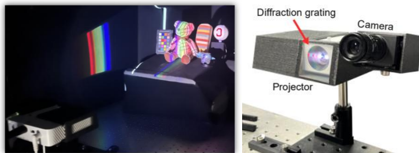
그림 1. CVPR 2024, Dispersed Structured Light for Hyperspectral 3D Imaging 이미징 시스템
