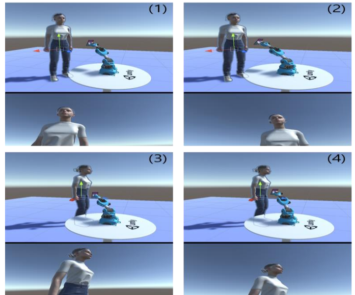
그림 3: 객체 탐지 모델을 이용한 얼굴 탐지 및 추적 1) 초기 상태, 2) 얼굴을 인식하고 화면 중앙에 위치하도록 로봇을 이동, 3) 사용자가 새로운 위치로 이동, 4) 새로운 위치에서 발견된 얼굴이 중앙에 위치하도록 이동
