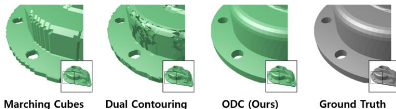
그림 2. 추출된 메쉬 비교. ODC의 결과가 기존 방법 대비 sharp feature를 가장 잘 보존한다.
