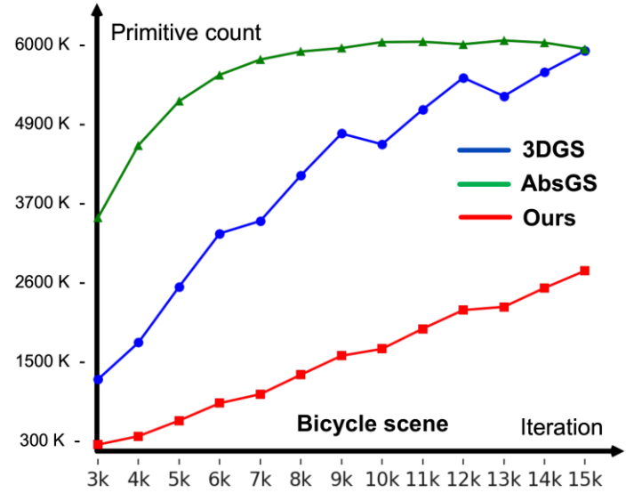
그림 3 Primitive 수 변화
