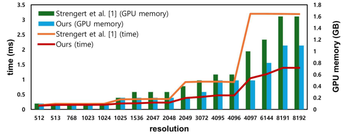
그림 3: 이미지 해상도별 인페인팅 속도와 GPU 메모리 사용량 비교 결과
