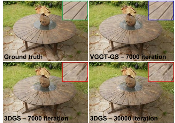
그림 3 Qualitative Comparison under 24-view setup
