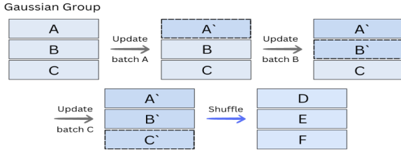
그림 2: 배치별 가우시안 업데이트
