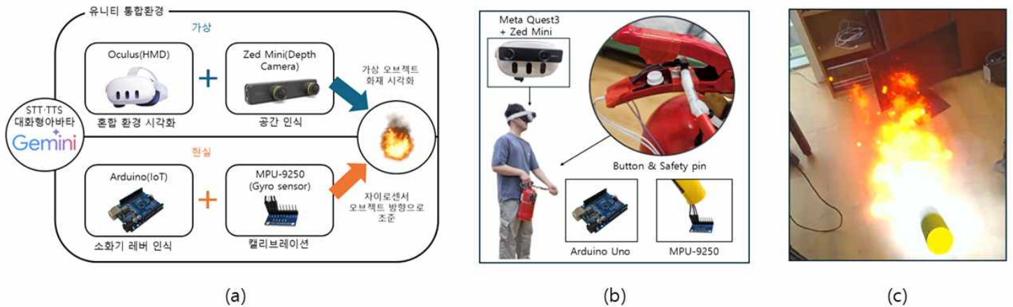
그림 1: 실가상 통합 소방 훈련 시스템, (a) 시스템 아키텍처, (b) 주요 하드웨어 구성, (c) HMD 시뮬레이션 화면
