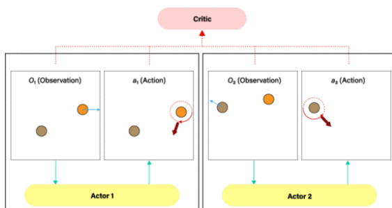
그림 1. 여러 사용자의 리셋 방향을 학습하는 MARR 모델 개요도
