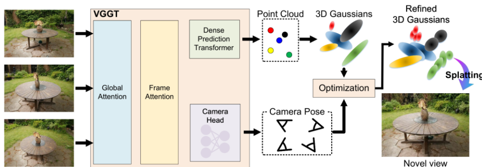
그림 1 Overview of VGGT-based Initialization for 3D Gaussian Splatting
