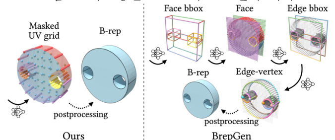
그림 2. BrepDiff의 전체 구조와 다단계구조인 BrepGen[1]의 전체 구조
