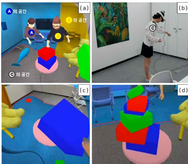
그림 2: (a) 사용자 C 관점에서 사용자 A, B의 아바타와 공간이 함께 보이는 모습 (b) 실제 공간에서 시스템 체험 중인 사용자 C의 모습 (c) 조각이 공간 내에 흩어져 있는 초기 모습 (d) 공간 내의 조각을 협력하여 모두 찾아 답을 완성한 모습
