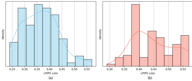
그림 2. LPIPS 손실 분포 (a)는 픽사 스타일, (b)는 지브리 스타일에 대한 LPIPS 손실의 분포.
