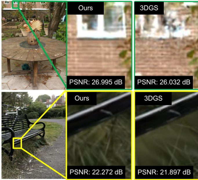
그림 2 시각적 비교
