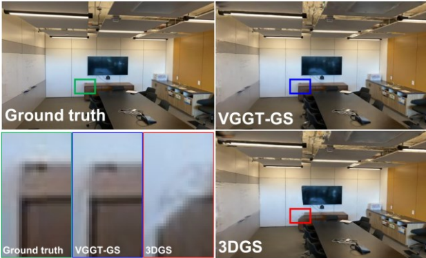
그림 2 Qualitative Comparison under full-view supervision
