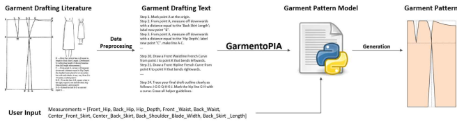
그림 2: GarmentoPIA를 이용한 의복 패턴 생성 절차
