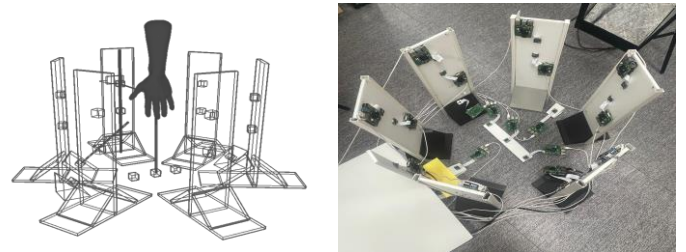
그림 1: 스캔 시스템 구조 설계도 및 구현 사진
