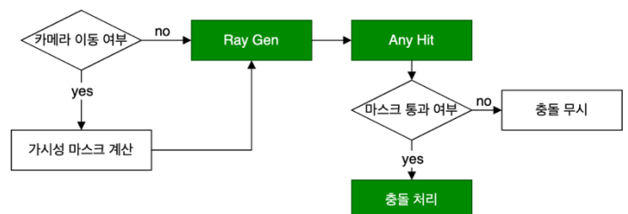
그림 1. 3DGRT 렌더링 파이프라인 내 가시성 마스크 삽입
