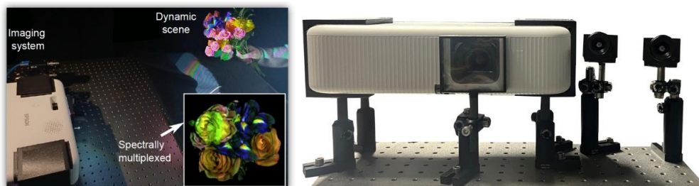
그림 2. CVPR 2025, Dense Dispersed Structured Light for Hyperspectral 3D Imaging of Dynamic Scenes 이미징 시스템
