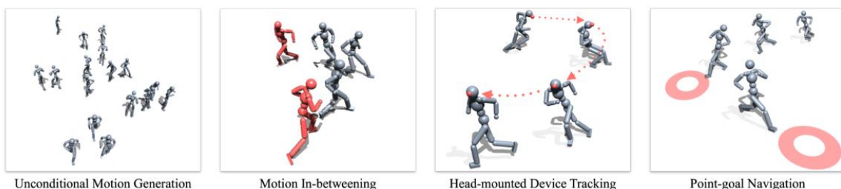
그림 2. 다양한 작업에 재사용 가능한 모션 사전 지식 학습
