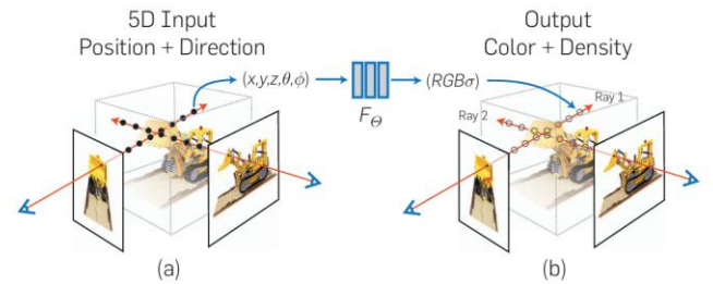
그림 1: NeRF[1]의 학습 과정
