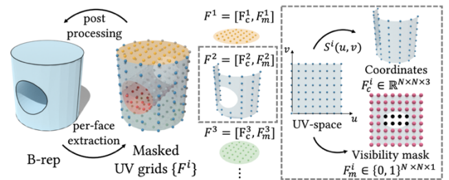
그림 1. 마스킹된 UV 그리드 표현의 예시.
