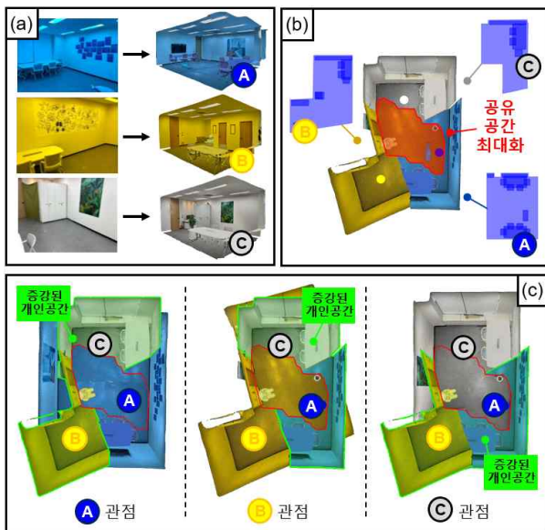
그림 1: 시스템 개요 (a) 사용자 A, B, C의 물리적 실공간의 디지털 카피 (b) 사용자 A, B, C의 공간에서 2D 평면도를 추출하여 공유 공간을 최대화하는 방식으로 정렬시킨 모습 (c) 사용자들의 위치에 따라 각자의 개인 공간의 보여지는 범위가 결정된 동일한 순간의 사용자 A, B, C 관점
