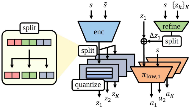
그림 1: 부위별 잠재 토큰 및 정책 네트워크
