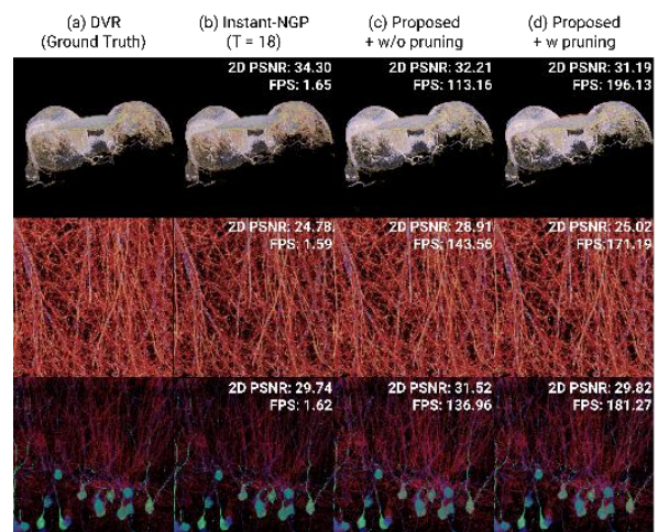
그림 2. 3D Gaussian Splatting을 통한 볼륨 경량화 결과
