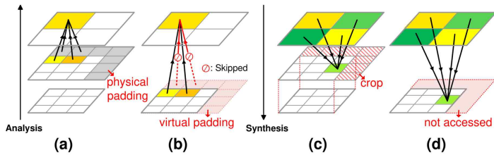
그림 2: 기존 방식 (a), (c)의 물리적 패딩과 제안 방식 (b), (d)의 가상 패딩을 적용한 분석 및 합성 과정 비교.
