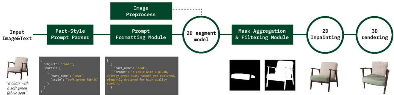
그림 2: 전체 파이프라인과 입력 처리 예시.
