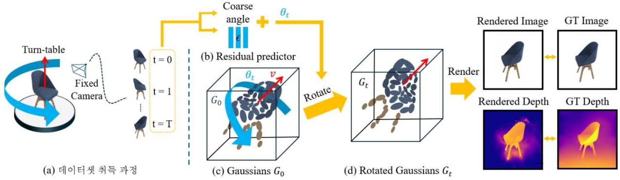
그림 1: 전체 파이프라인, (a) 고정된 카메라로 회전하는 원판 위의 물체를 촬영하여 최대 timestep T까지의 데이터를 취득한다. (b-d) 회전각이 0인 가우시안 집합 G_0 를 회전축 v 를 기준으로 회전각 \theta_t 만큼 회전시킨 가우시안 집합 G_t 를 렌더링한 결과와 ground-truth 사이의 손실값을 바탕으로 G_0 , v , 그리고 회전각 잔차 예측 모델의 변수 \epsilon 를 학습한다.
