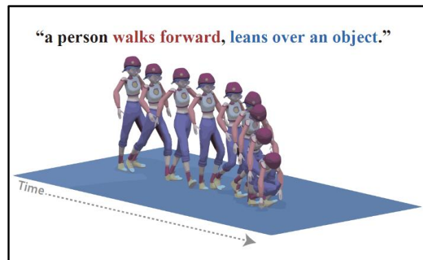
그림 2. Text-to-Motion 예시
