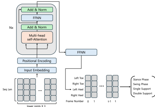
그림 3: 네트워크 구조
