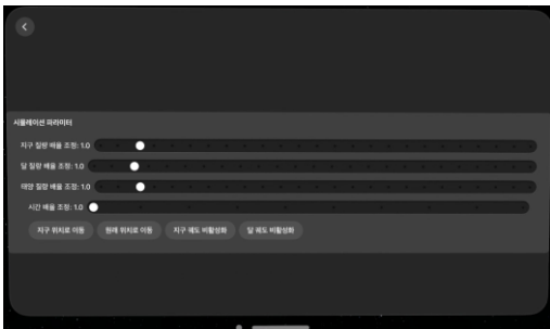
그림 2: UI창
