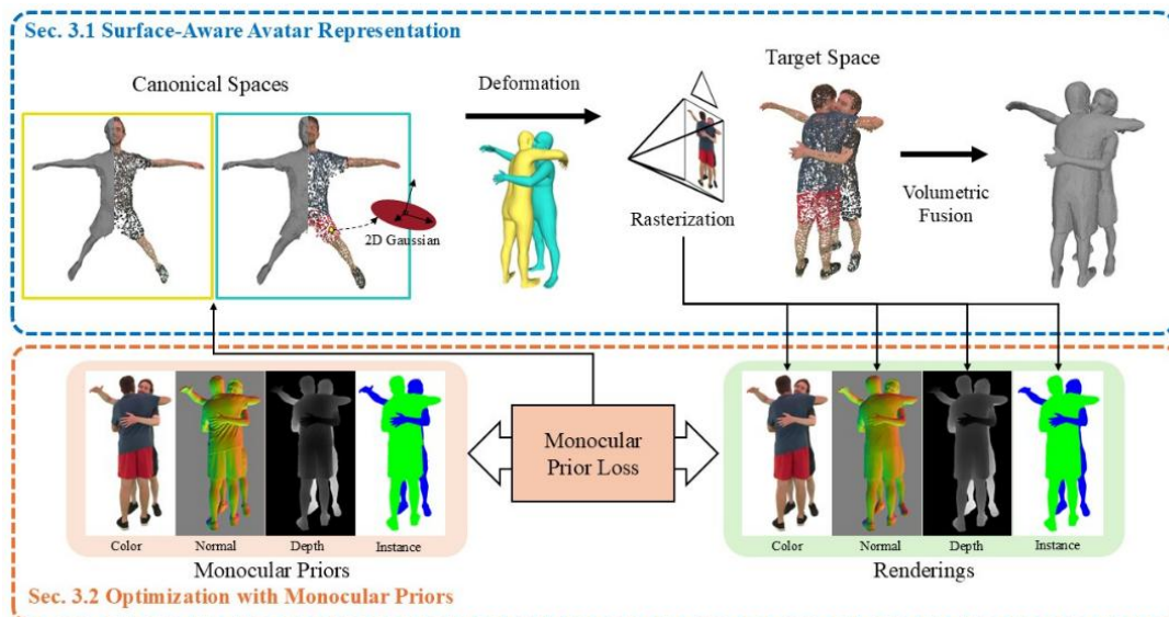
그림 1. GeoAvatar의 파이프라인
