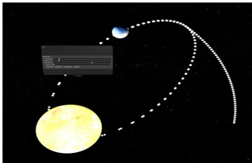
그림 3: 태양의 질량을 증가시켰을 때
