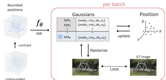
그림 1: 방법론 개요
