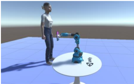
그림 1: 시뮬레이션 환경
