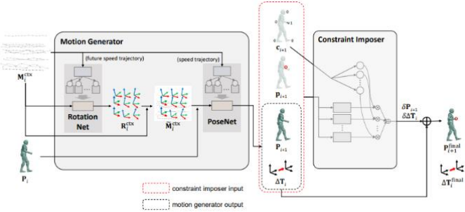
그림 2: 네트워크 Overview
