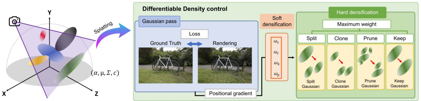
그림 1 미분 가능한 밀도 제어 기반 3DGS 개요도
